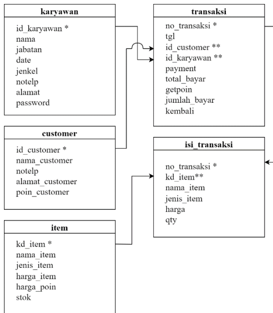
Gambar 4. Normalisasi
