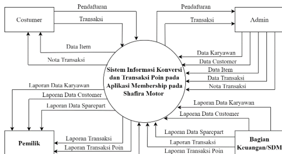
Gambar 2. Diagram Konteks
