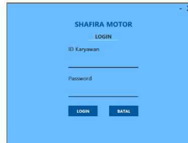
Gambar 6. Tampilan Login
