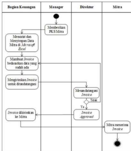
Gambar 1 Proses Sistem Berjalan
