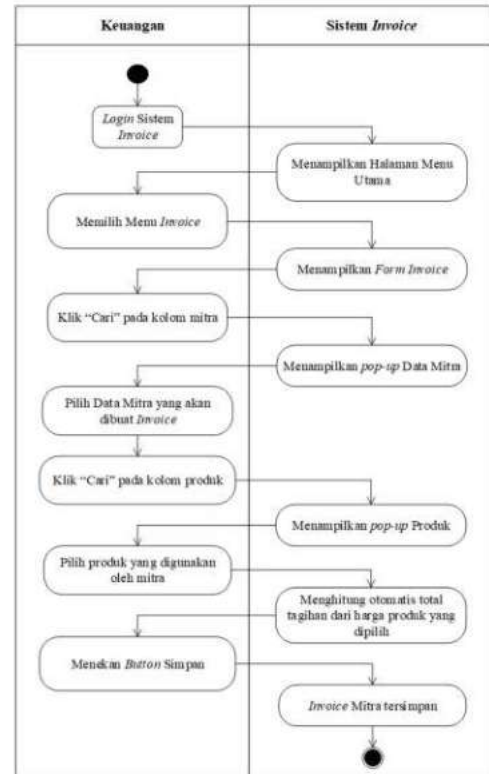
Gambar 3 Activity Diagram Pembuatan Invoice
